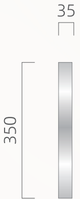
侧视图 SIDE
